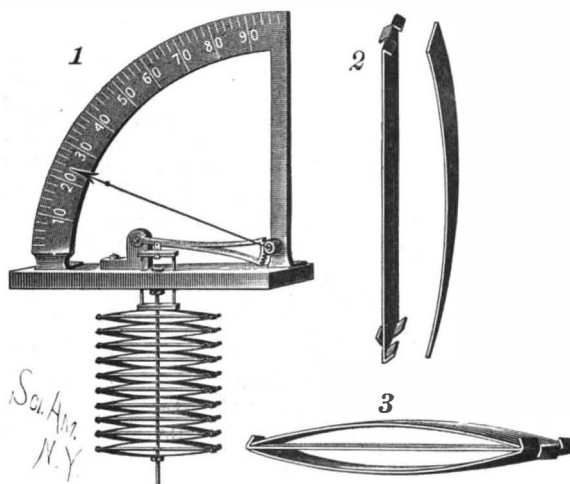
Fig. 2.—THERMOSTAT.
