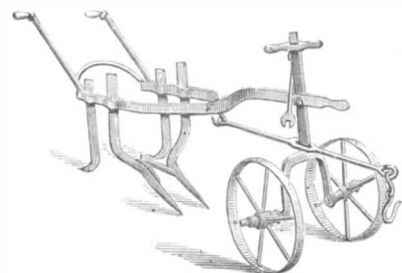
Fig. 30.—BEET-ROOT PULLER.
