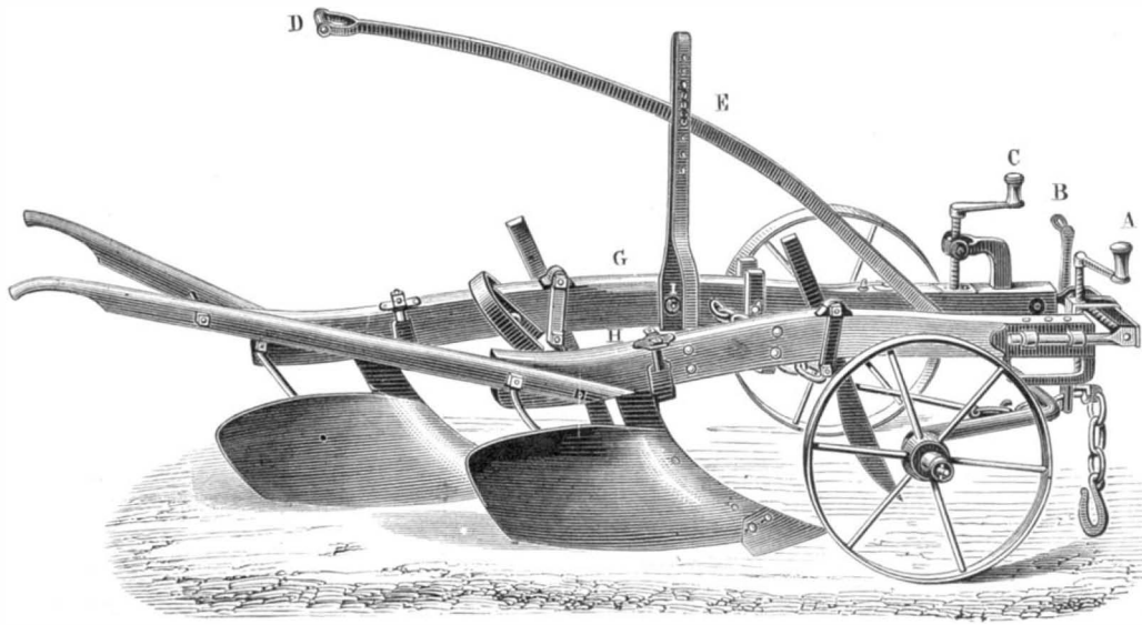
Fig. 18.—MEIXMORON-DOMBASLE'S BISOC.
